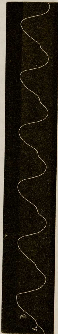
Fig. 85. — Tracé des pulsations du cœur chez une grenouille
