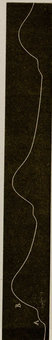
Fig. 86. — Tracé des pulsations du cœur chez une anguille.
