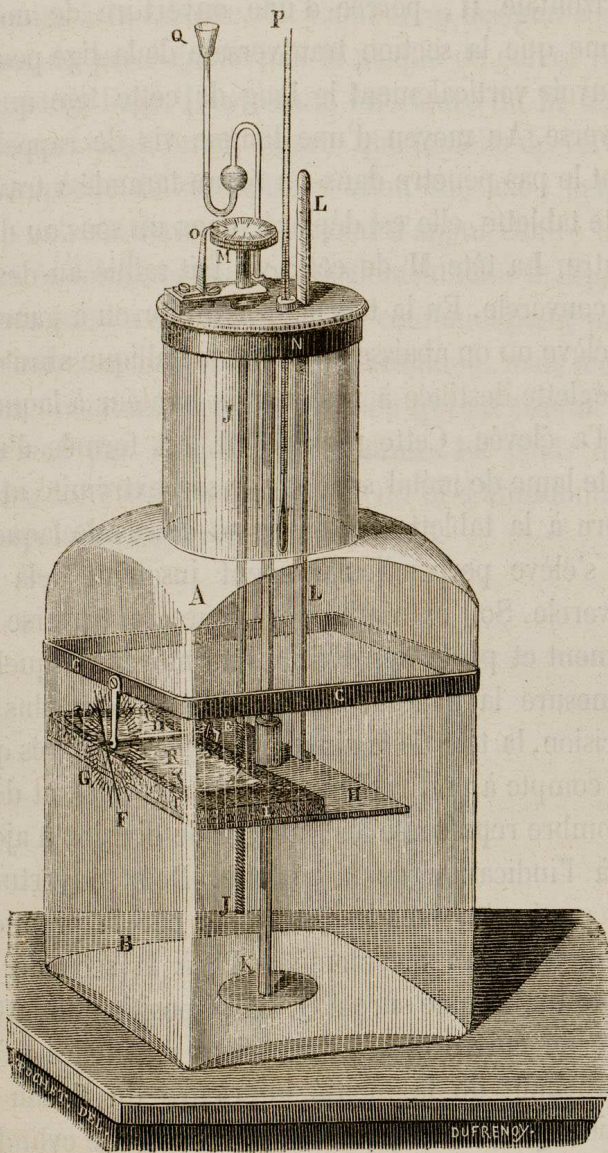
Fig. 32. — Appareil de M. Callibrucès pour mesurer les variations d'intensité des mouvements vibratiles.
