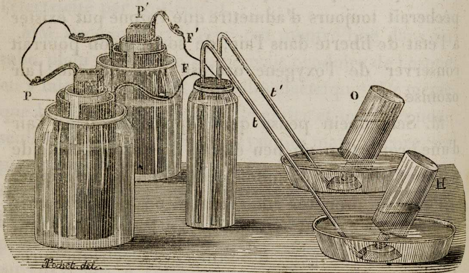
FIG. 7. — Appareil à produire de l'ozone.
