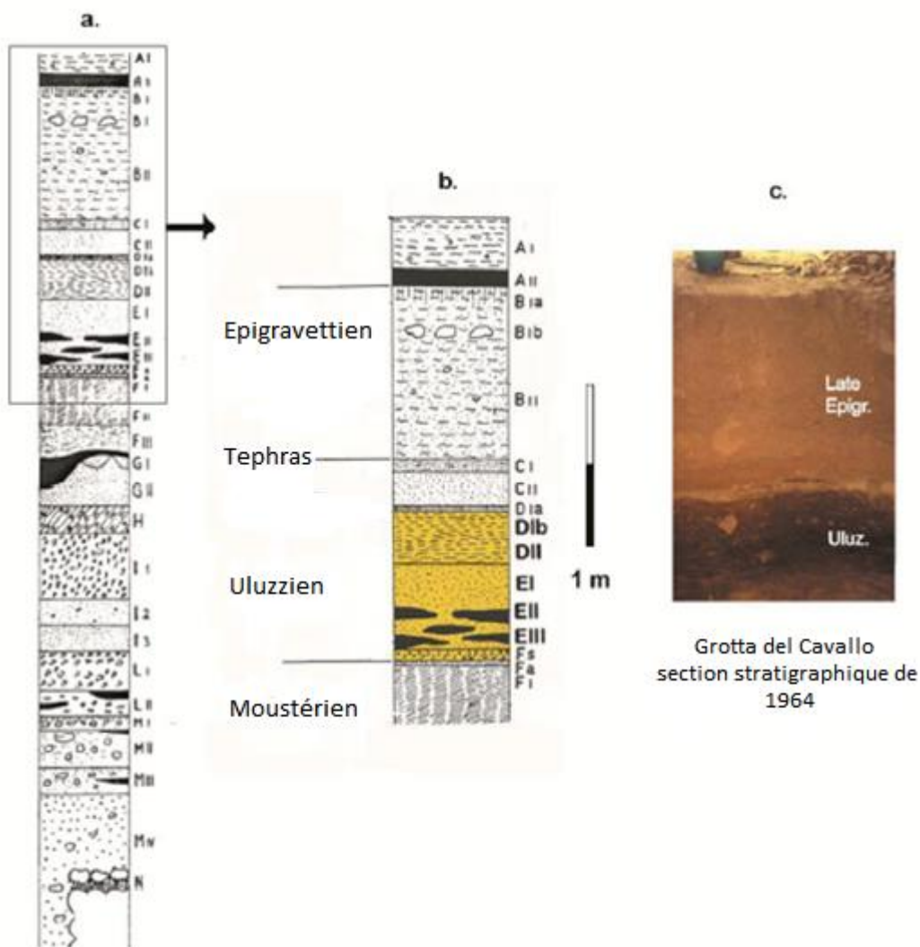
FIGURE 9 : Section stratigraphique de la période du paléolithique de la Grotta del Cavallo (d'après Benazzi et al., 2011). (n°30)
