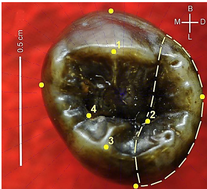
FIGURE 2 : Photographie occlusale d'une première prémolaire inférieure d' Homo erectus , avec positionnement de points-repères et construction de points glissants (d'après Gómez-Robles et al., 2008). (n°8)
