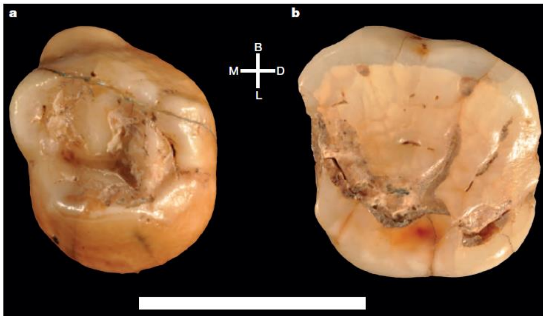
FIGURE 10 : Vue occlusale des molaires lactéales de la Grotta del Cavallo (d'après Benazzi et al., 2011) (n°13)
