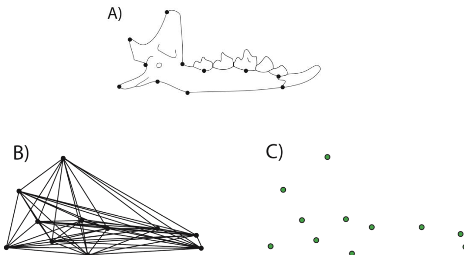
FIGURE 3 : Description en 2D de la géométrie d'une mandibule de Musaraigne, avec 11 points-repères (d'après Perrard, 2012). (n°5)
