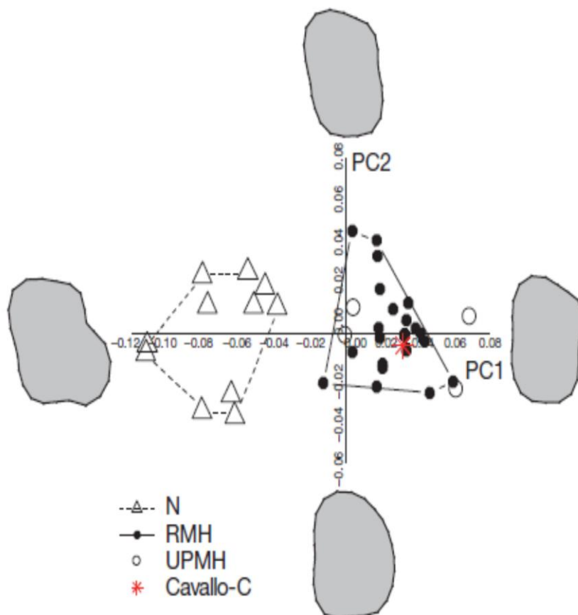
FIGURE 13 : Représentation graphique des différences de forme (contours cervicaux) des dM2 de l'échantillon (d'après Benazzi et al., 2011). (n°13)
