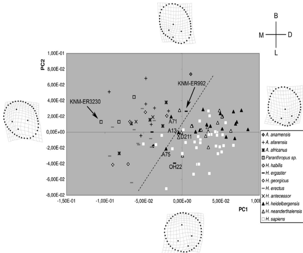
FIGURE 6 : Représentation graphique par PCA et TPS des différences de forme des premières prémolaires inférieures des différentes espèces d'homininés. (d'après Gómez-Robles et al., 2008). (n°8)
