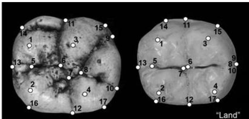
FIGURE 4 : Photographies occlusales de deux 2èmes molaires inférieures d'homininés, avec positionnement de 17 points-repères. (n°11)
