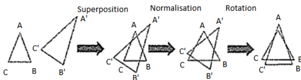
FIGURE 5 : Les étapes de la superposition Procruste (d'après Evin et al., 2008). (n°12)
