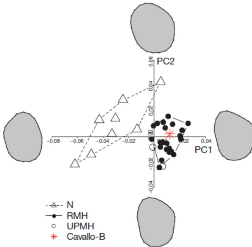
FIGURE 12 : Représentation graphique par PCA des différences de forme (contours coronaires) des dM1 de l'échantillon (d'après Benazzi et al., 2011). (n°13)
